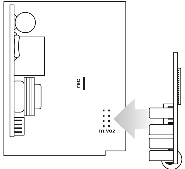
Módulo Discador MD8
